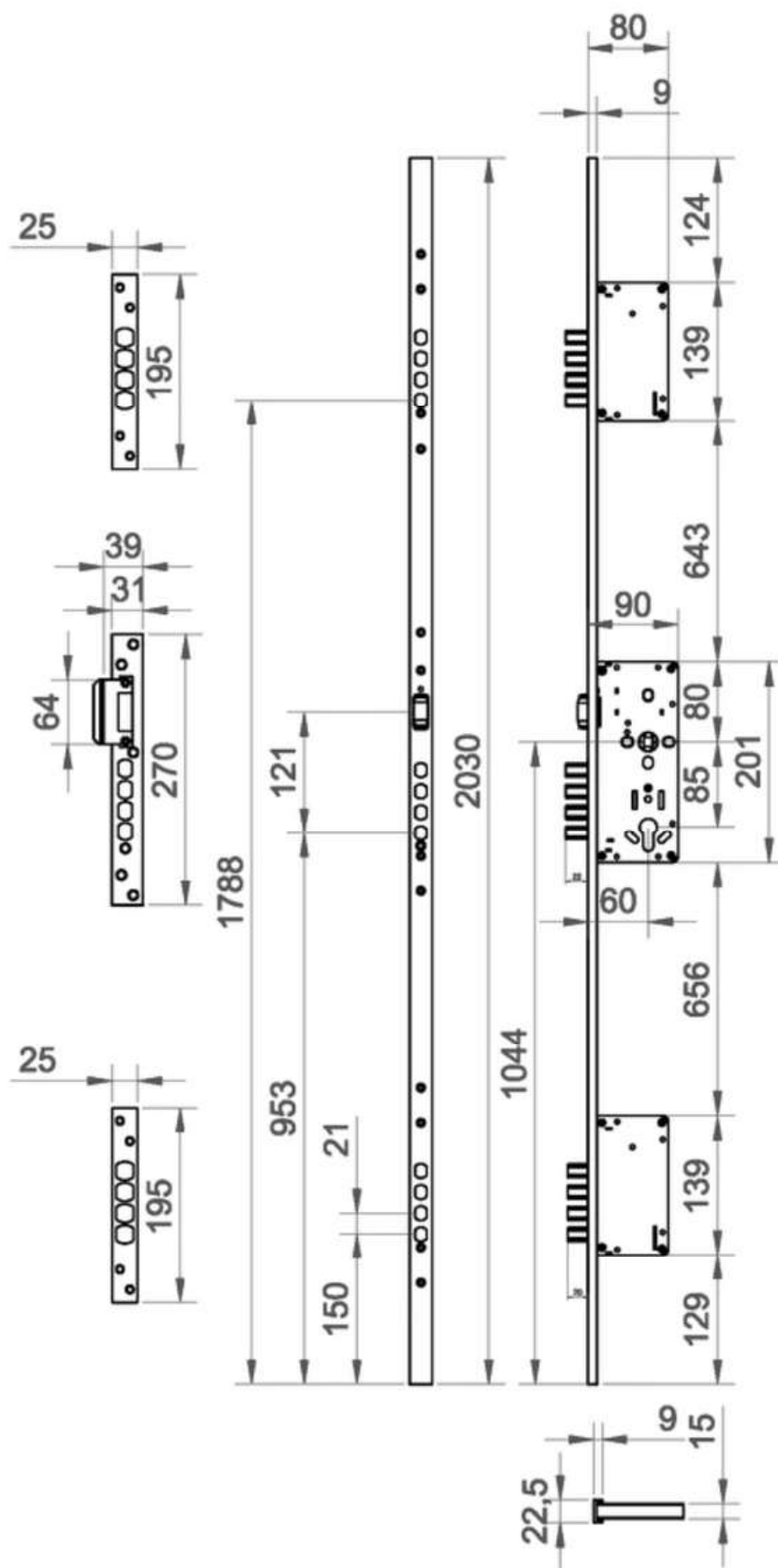
FECHADURA TIPO MULTIPONTO 70200
