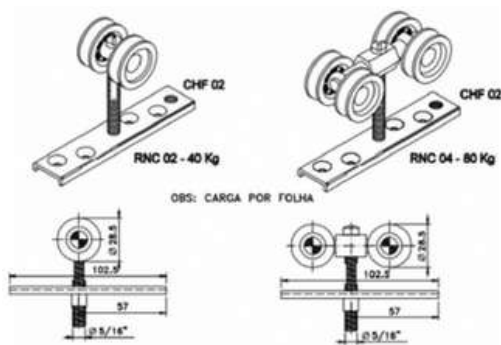
ROLDANA ROL RRC02 OU RRC 04
