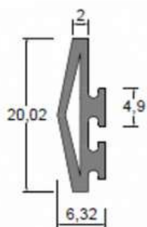
GUA-ACM01 - BSB 1124 CORDÃO EM EPDM PARA PORTAS EM AC
