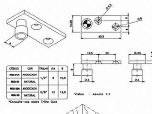
ROLETE GUIA RU
